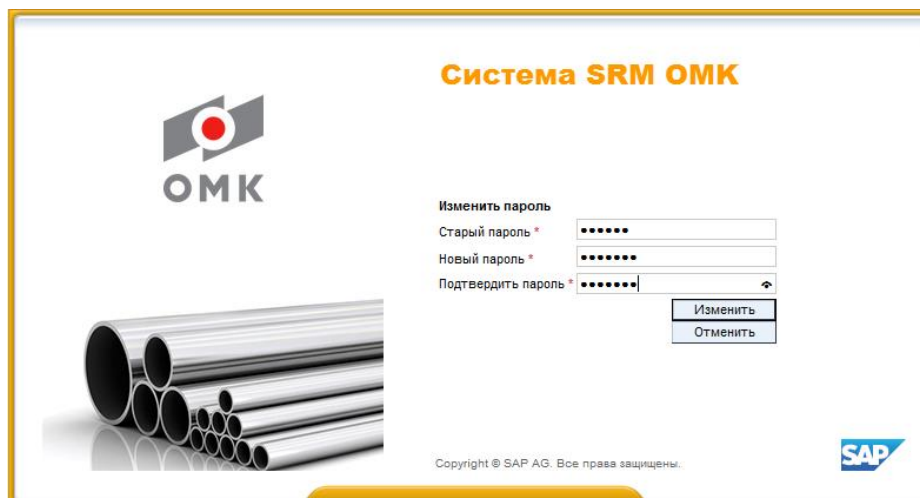
Рисунок 2 – Смена пароля
