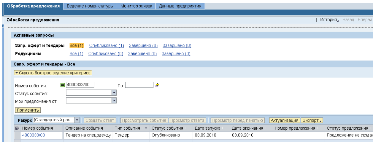
Рисунок 10– Обработка предложения
